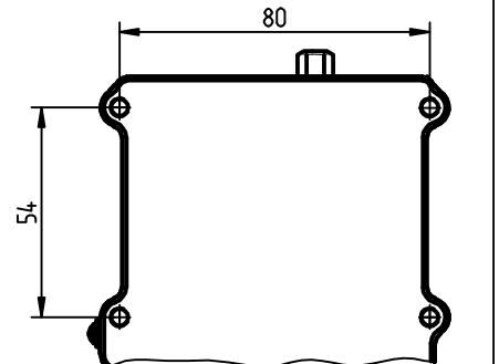
А (1:2) Габариты крепежных отверстий
